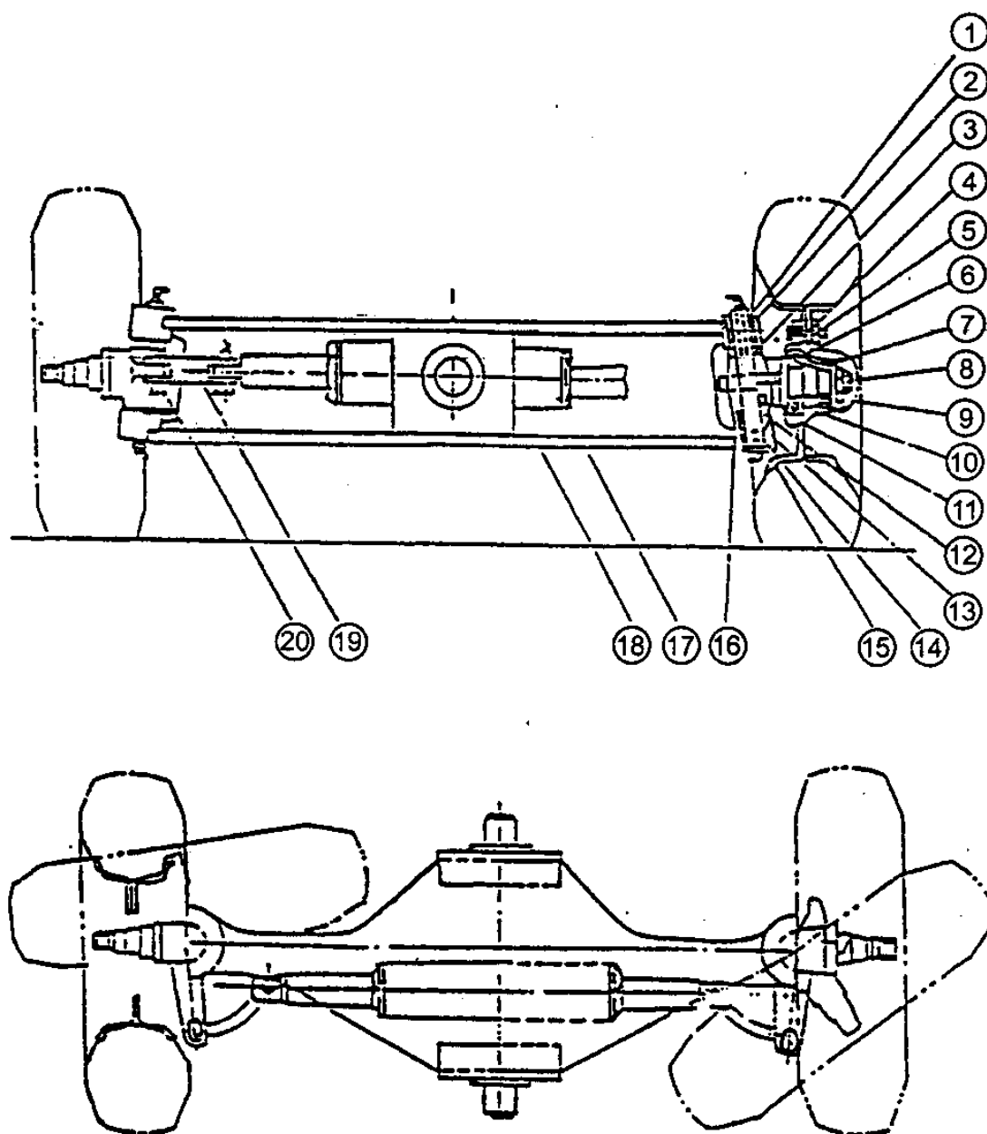
рисунок 3-3 рулевая ось
