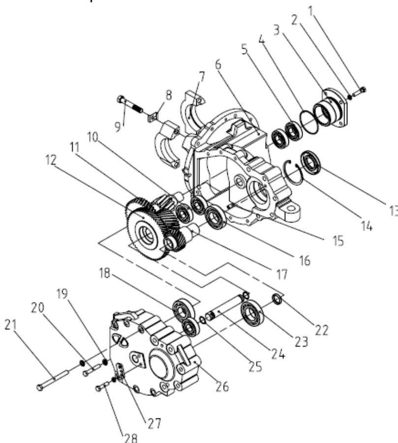
Рис. 1-1 Редуктор понижающей передачи
