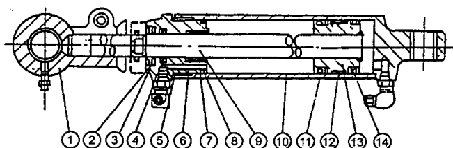
рисунок 7-8 цилиндр наклона
