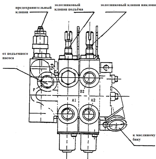
рисунок 7.1 регулирующий клапан
