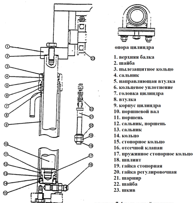
рисунок 7-4 подъемный цилиндр
