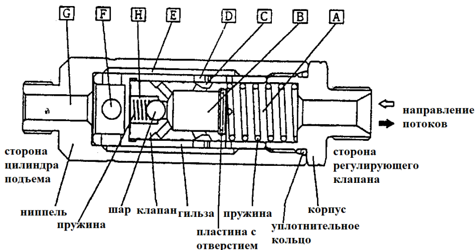
рисунок 7-7 клапан регулятора расхода
