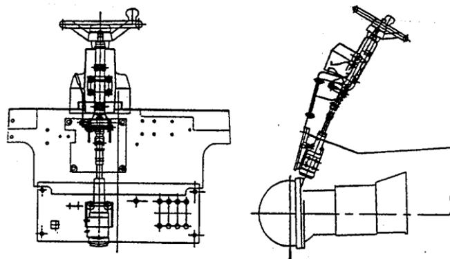
рисунок 3-1 рулевая система
