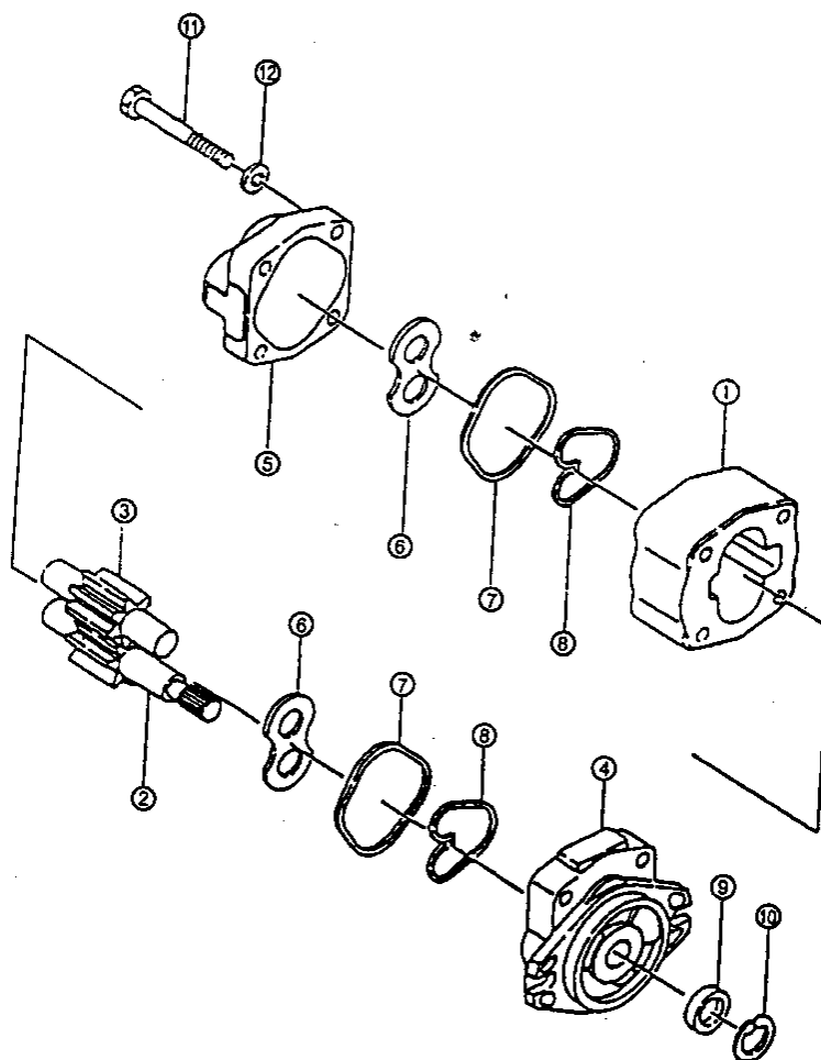
рисунок 7-16 шестерёнчатый насос
