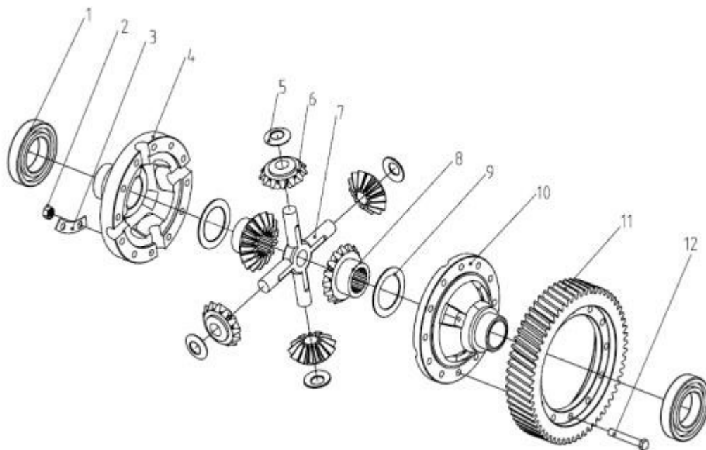
Рис. 1-2 Дифференциал
