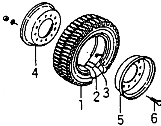
рисунок 3-7 сборка колеса
