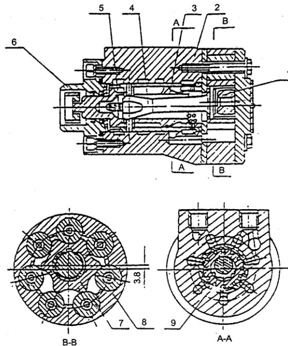
рисунок 3-2 циклоидная передача тип рулевого управления
