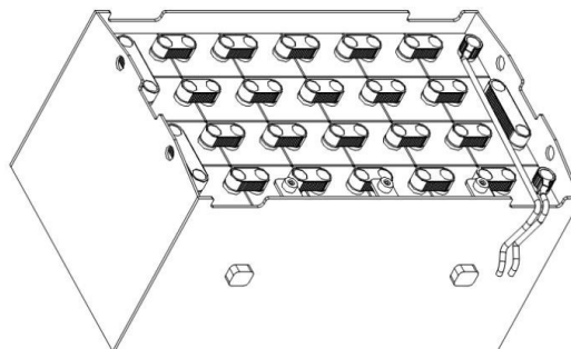
Рис. 6-1 Аккумулятор
