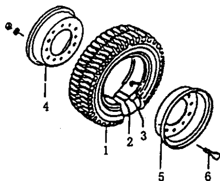
1-6 рисунок. колесо в сборе
